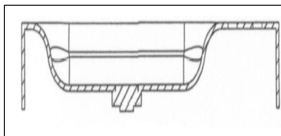
Zapsaný průmyslový vzor Beneluxu č. 38478-0002 (23.02) (umyvadla), majitel: Maan Amsterdam Holding BV
